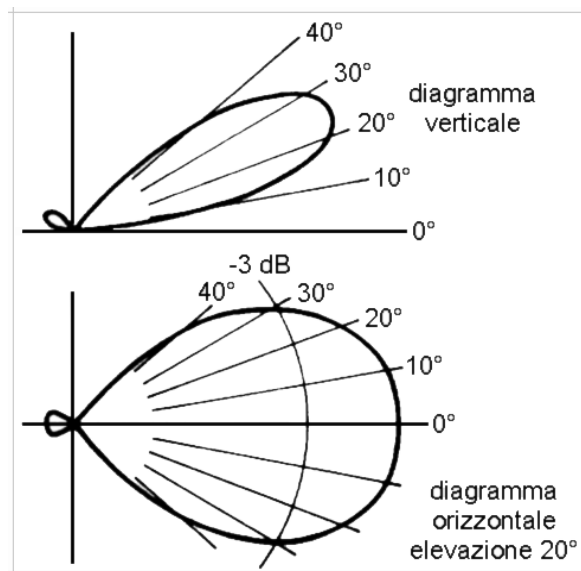
Diagrammi d'irradiazione di una Yagi a tre elementi distante dal suolo L \frac{1}{2} (mezzi)
